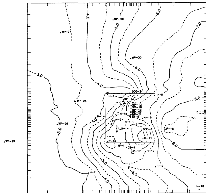
A. KRIGED TRANSMISSIVITIES
